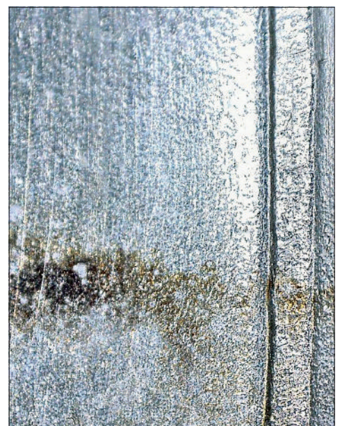
Abb. 11: Ausführung CC, Korrosion am Flüssigkeitsspiegel
