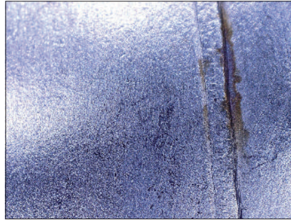
Abb. 7: Ausführung CC, Schweißnahtkorrosion
