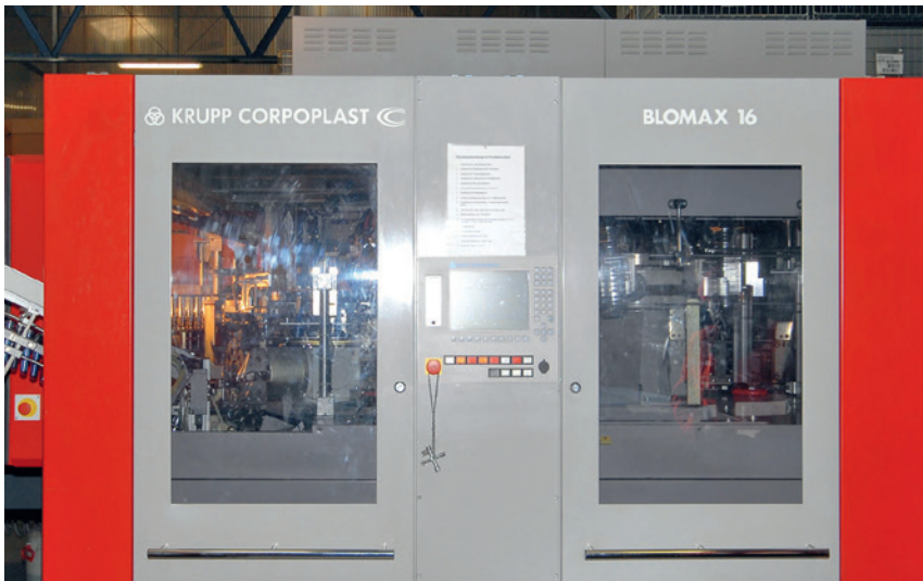
Streckblasmaschine – neue Generation führt zu hoher wirtschaftlicher Abnutzung
